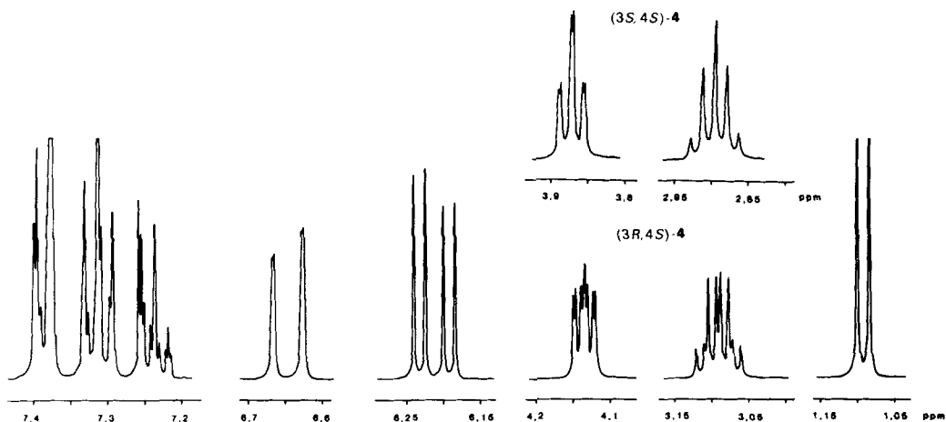
Fig. 1. 400-MHz- 1 H-NMR-Spektrum (CDCl 3 ) von (3 R ,4 S )- 4 und die wichtigsten davon abweichenden Signale von (3 S ,4 S )- 4
