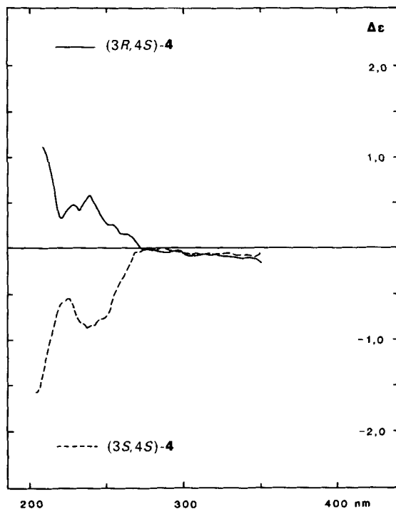
Fig. 2. CD-Spektren (0,01 N HCl) von (3 R ,4 S )- 4 und (3 S ,4 S )- 4
