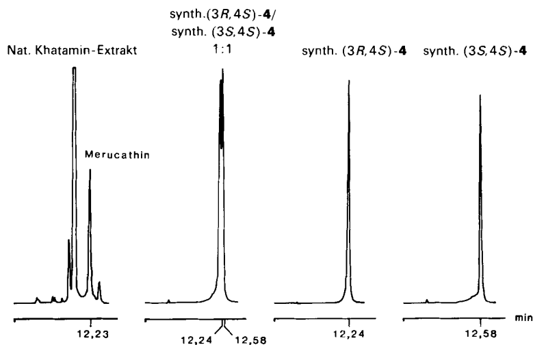
Fig. 3. HPLC-Trennung eines natürlichen Khatamin-Extraktes im Vergleich mit den beiden synthetisierten Verbindungen (3 R ,4 S )- 4 und (3 S ,4 S )- 4 . Lichrosorb Si 60 5 \mu m. CH 2 ClCH 2 Cl/MeOH/AcOH/H 2 O/Et 2 NH 800:200:10:5:5 v/v, 0,8 ml/min. Detektion bei 254 nm [3].
