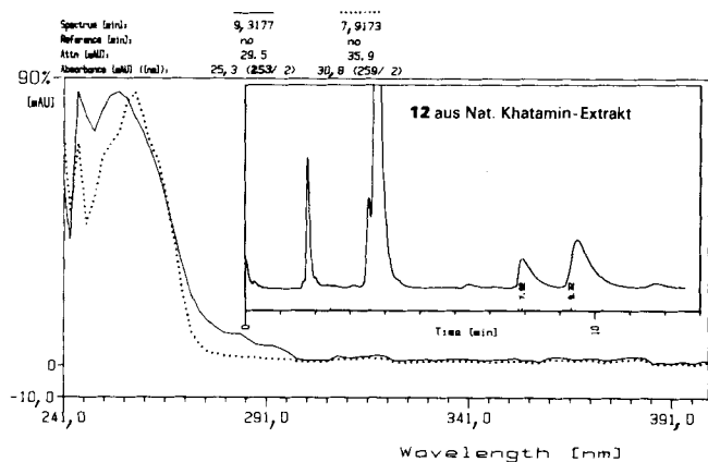
Fig. 4. HPLC-Trennung und Diodenarray-Spektrophotometrie von nach [18] hergestellten ( 1'S,2'R,1''R )-12 und ( 1'R,2'S,1''R )-12 und Vergleich mit den aus einem natürlichen Khatamin-Extrakt erhaltenen Harnstoff-Derivaten 12 zur Zuordnung der abs. Konfiguration des natürlichen Merucathins. Gleichzeitige Bestimmung der optischen Reinheit von synthetischem ( 3R,4S )-4. Lichrosorb Si 60 5 \mu m, Hexan/ AcOEt 1:2, 1 ml/min. Detektion bei 254 nm.
